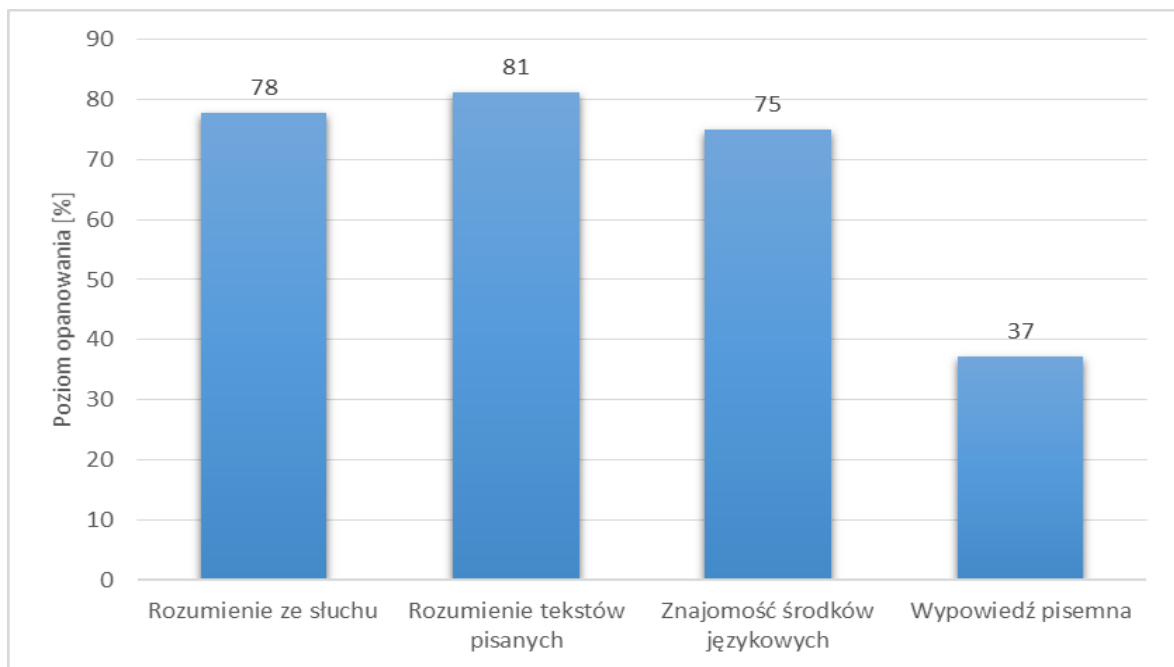
Wykres 2. Średnie wyniki zdających w zakresie poszczególnych obszarów umiejętności (dane krajowe)
